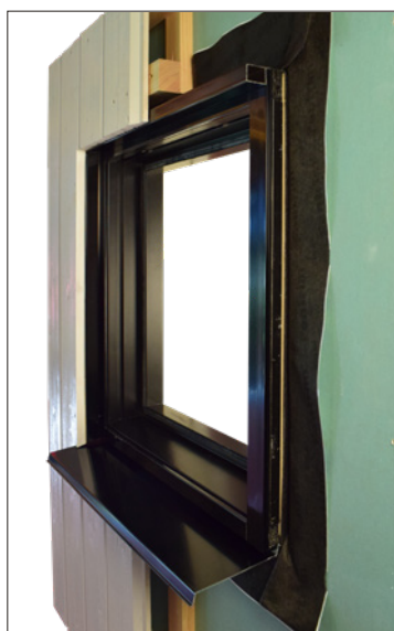
UTVENDIG FORINGSLIST
