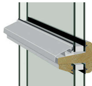
GJENNOMGÅENDE HORIZONTAL SPROSSE - UTSIDE
